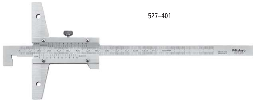
L 1 = Leitura no nônio de profundidade
